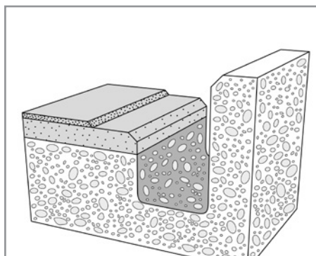
Fig 3.3.10. Rebaje en canalón
