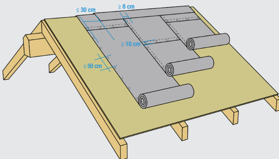
Fig 4.3.6. Fijación mecánica de láminas en pendientes mayores a 50%
