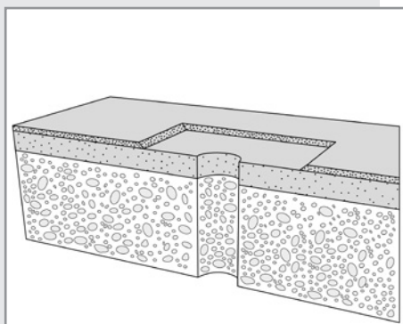
Fig 3.3.9. Rebaje en sumideros
