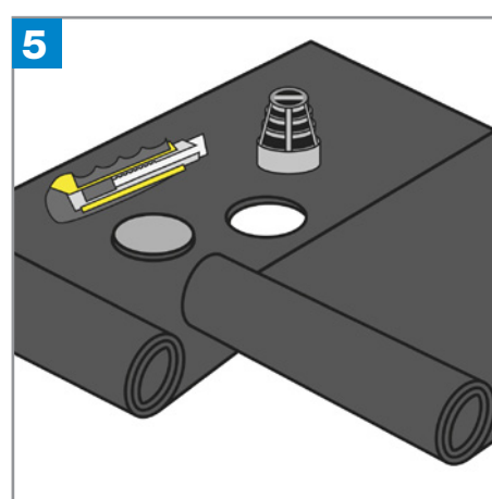
Fig.3.5.1. Desarrollo de sumidero vertical
