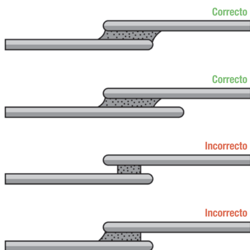
Fig. 4.3.4.1 Soldadura correcta.
