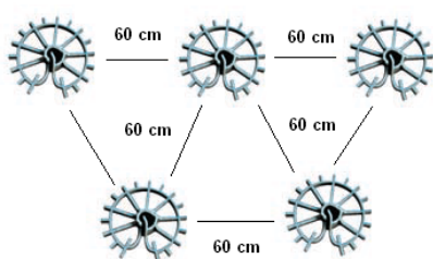
ESQUEMA DE COLOCACIÓN EN EL CORRUGADO
