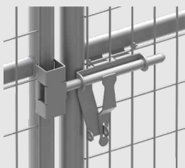
Cerrojo IT Detalle cerrojo y cerradero
