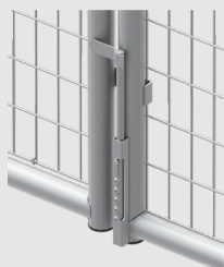
Pestillo de suelo IT Detalle pestillo de suelo
