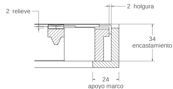
Detalle C
