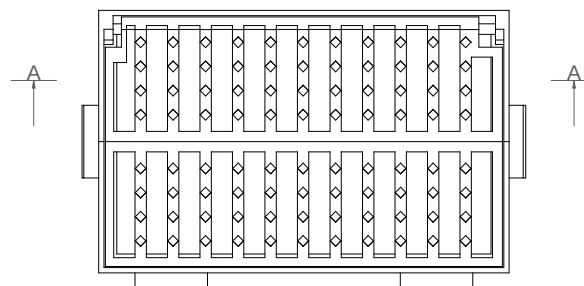
vista en planta 1:10
