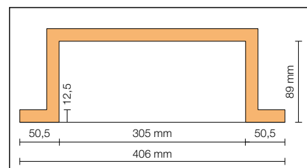
Schlüter®-KERDI-BOARD-N /-NLT
