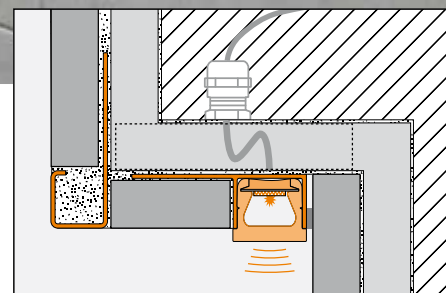
Schlüter®-KERDI-BOARD-NLT
